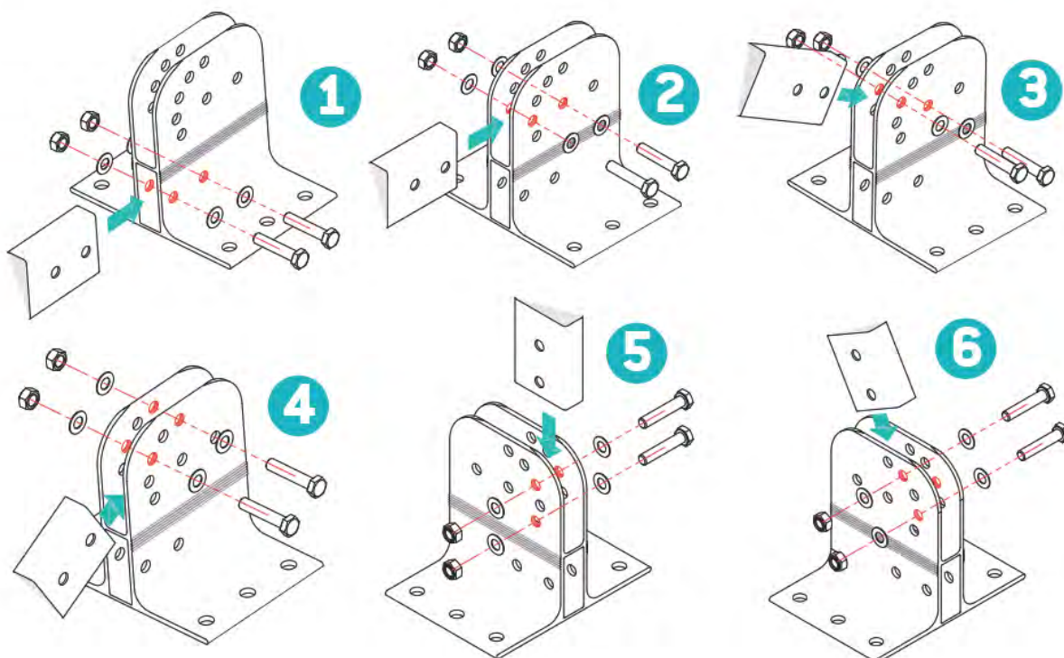
01 - RADENTE A PARETE 02 - DISTANZIATO 80 mm A PARETE 03 - A PARETE INCLINATO INTERNO 04 - A PARETE INCLINATO ESTERNO 05 - IN PIANO 06 - IN PIANO INCLINATO
