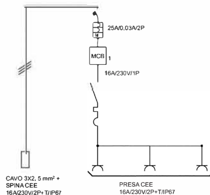
SCHEMA ELETTRICO COD. 40480
